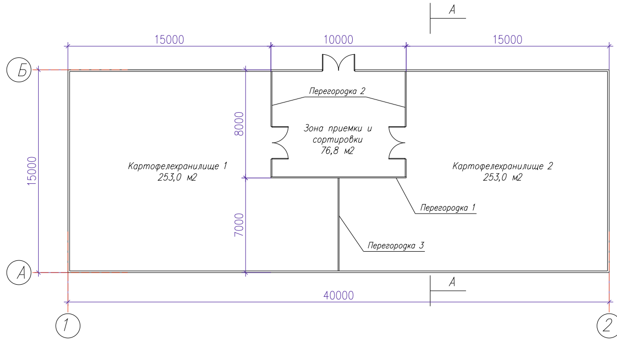
План картофелехранилища
