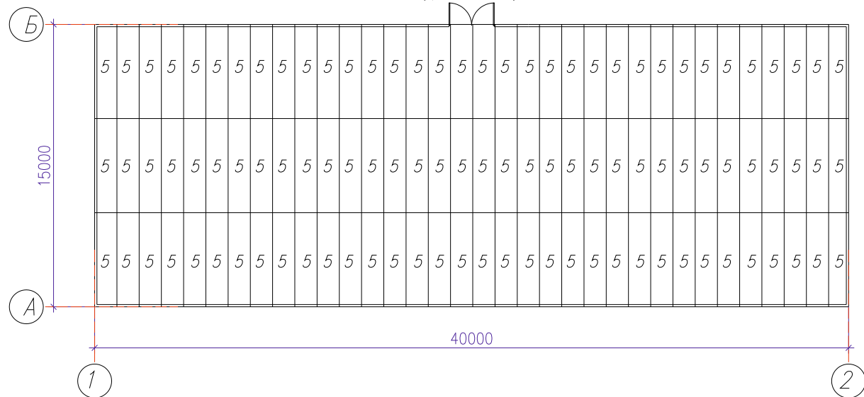
Схема раскладки стеновых сэндвич-панелей по полу/потолку
