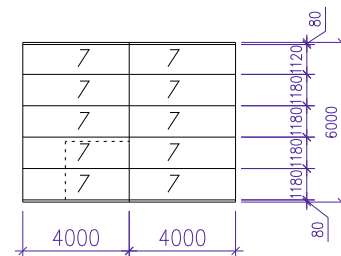
Схема раскладки стеновых сэндвич-панелей перегородка 2 (2шт)
