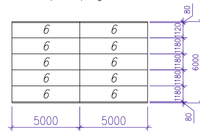
Схема раскладки стеновых сэндвич-панелей перегородка 1
