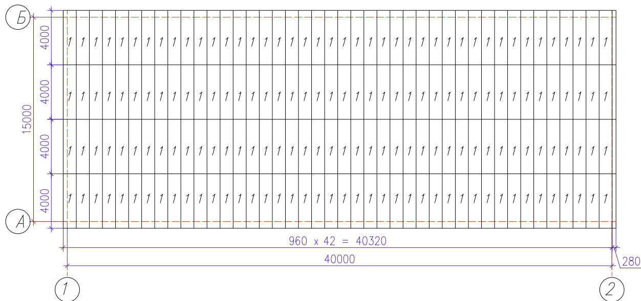
Схема раскладки кровельных сэндвич-панелей
