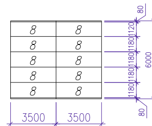
Схема раскладки стеновых сэндвич-панелей перегородка 3
